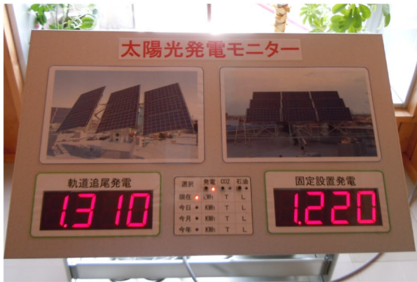
太陽光発電モニター(データロガー機能用)
